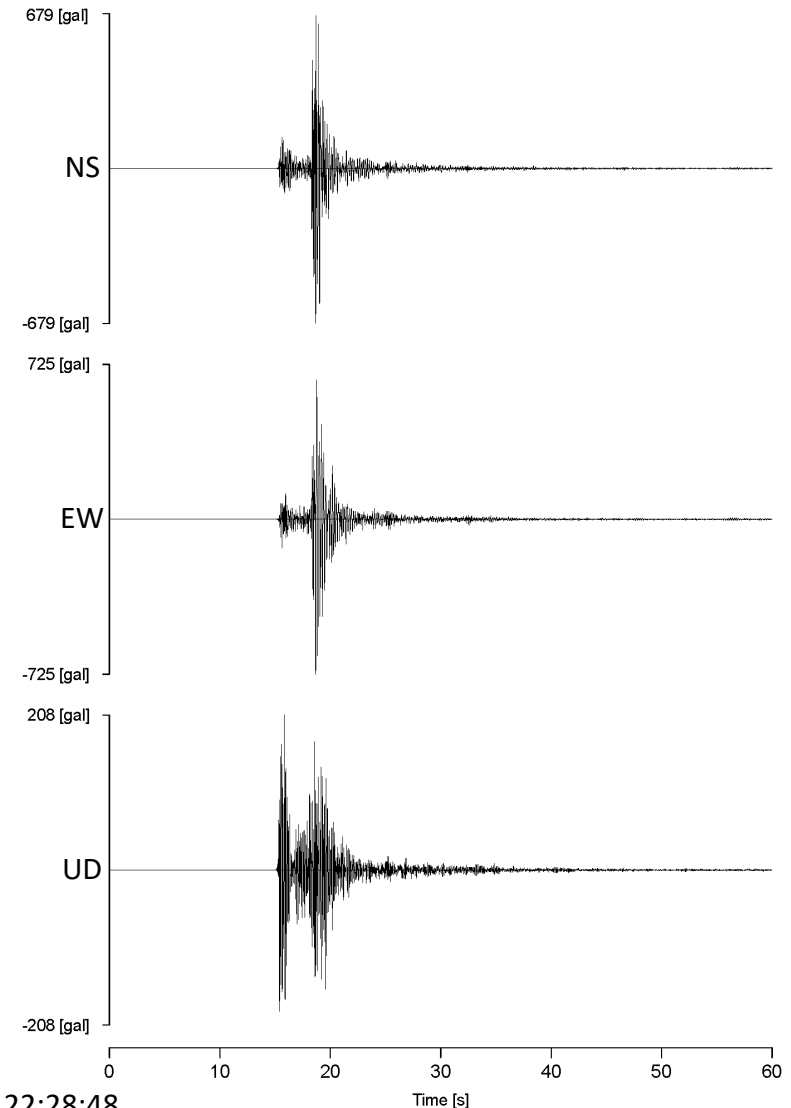
K-NET大月での加速度波形
