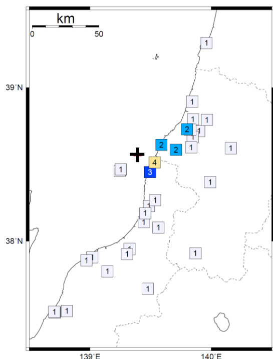
図3-2 19日00時57分 新潟県下越沖の地震 (M4.2、深さ12km、最大震度4)の震度分布図 (十印は震央を表す。凡例は図3-1と同様。)
