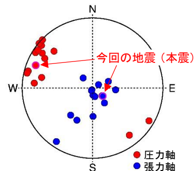
図2-8 領域b内の発震機構の 圧力軸と張力軸の分布
