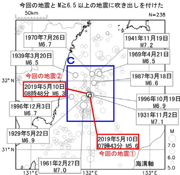
震央分布図 (1922年1月1日～2019年5月31日、 深さ0～100km、M \geq 5.0) 2019年5月の地震を濃く表示 今回の地震とM \geq 6.5以上の地震に吹き出しを付けた
