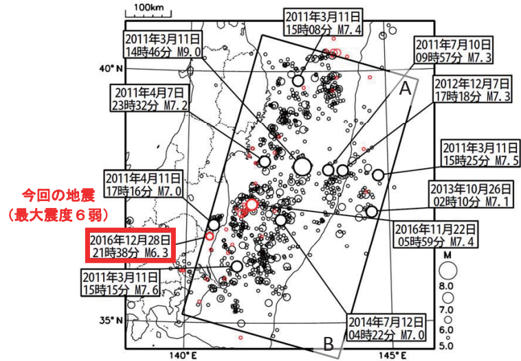
震央分布図
