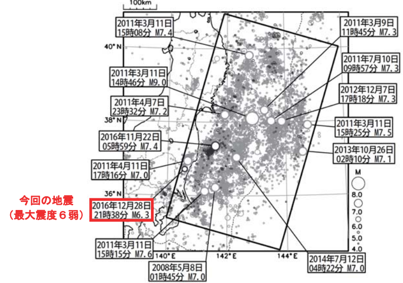
震央分布図
