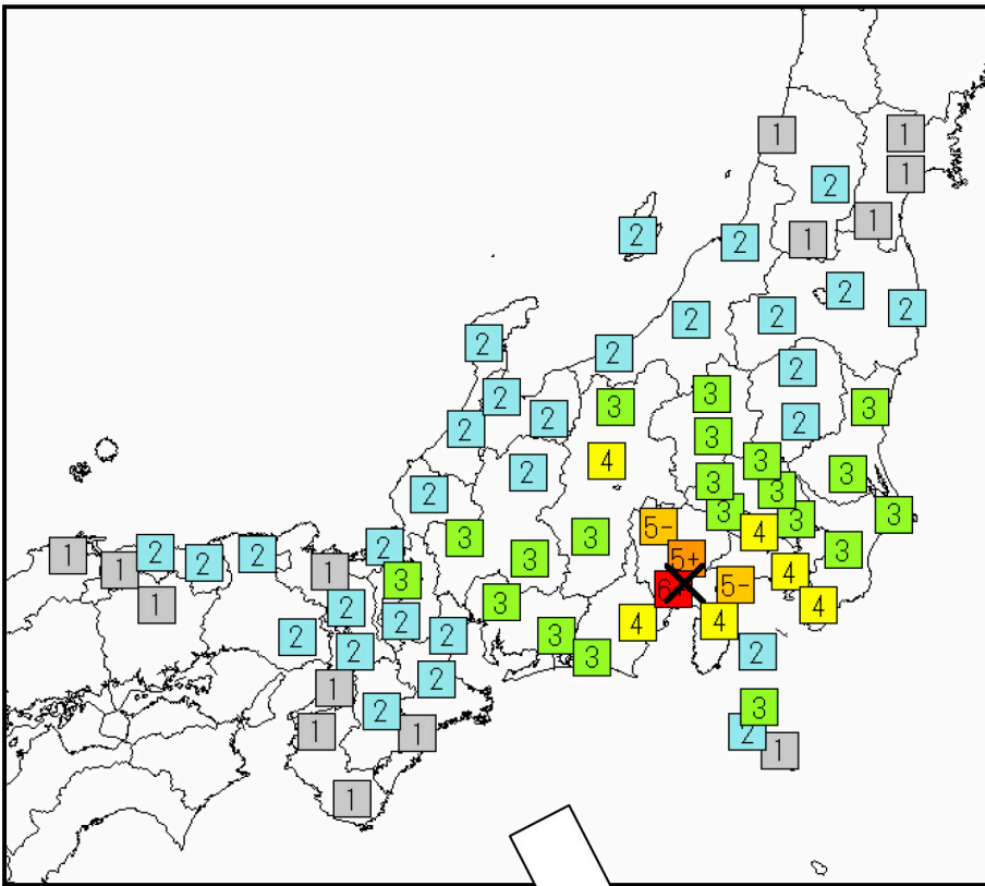
震度分布図
