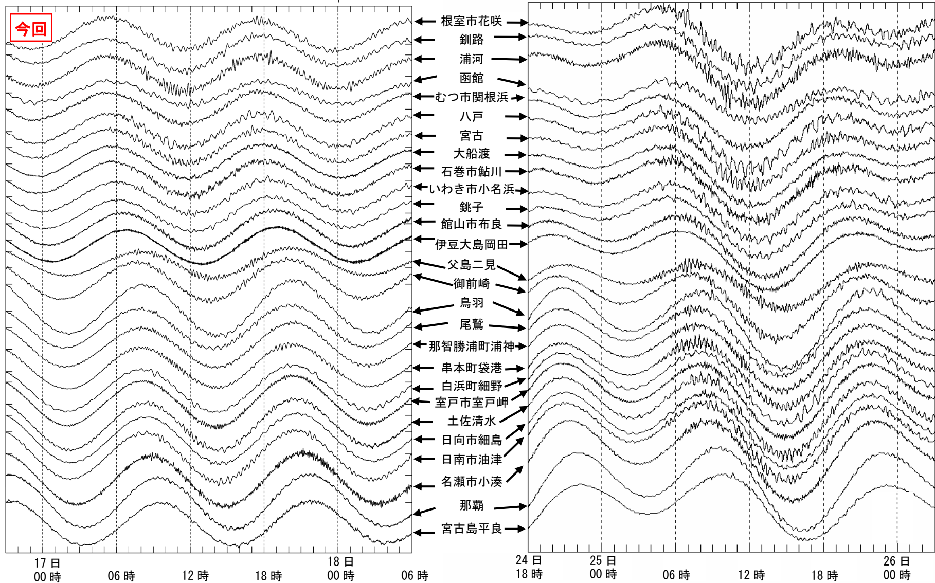
図 検潮所で観測した津波の波形比較
