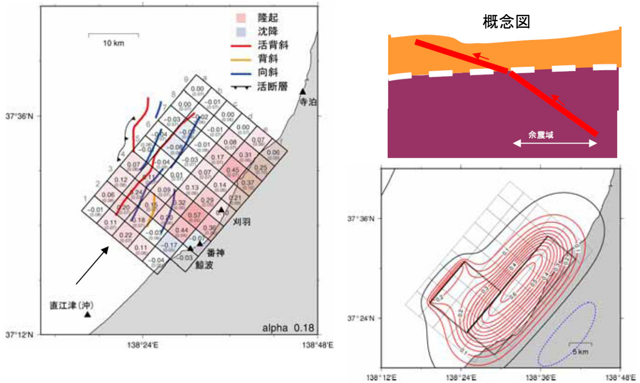
図 左) 岡村他 (2008) による背斜軸・向斜軸・活断層の位置と海底上下変動の比較。右) 南側・海側の隆起 (0.2m 程度) を説明するための南東傾斜断層モデル
