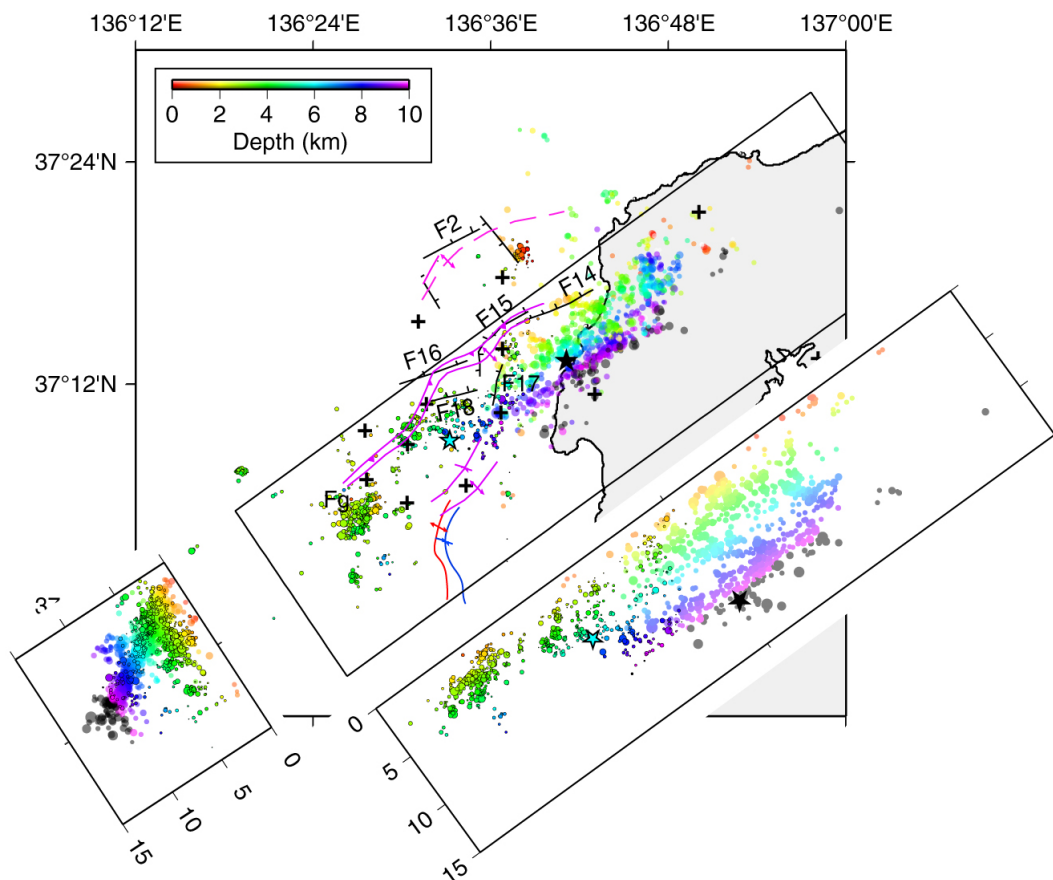
図 陸域には陸上臨時観測震源，海域に海底観測震源を用いた震源分布．海底観測震源には，丸の周囲を黒線で示してある．震源の色は深さを表す．黒い星印は，陸上臨時観測により，再決定された本震の震源位置，青い星印は，海底観測の結果を用いて，再決定された海域で発生した最大余震（3月26日7:16，M5.3）の位置．
