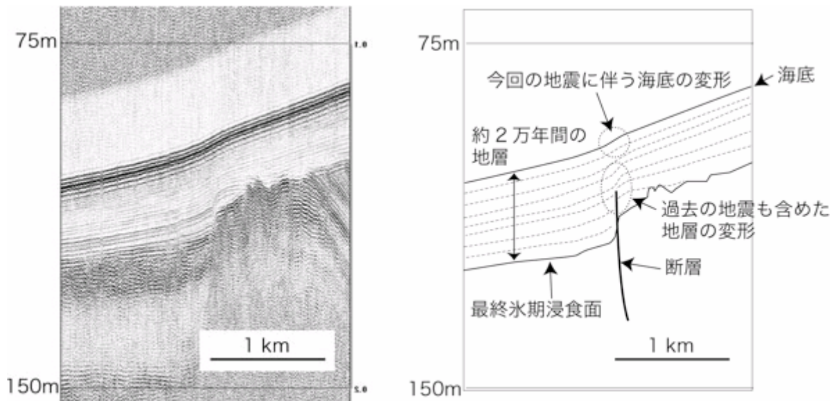
音波探査断面の実例（左）とその解釈断面（右）
