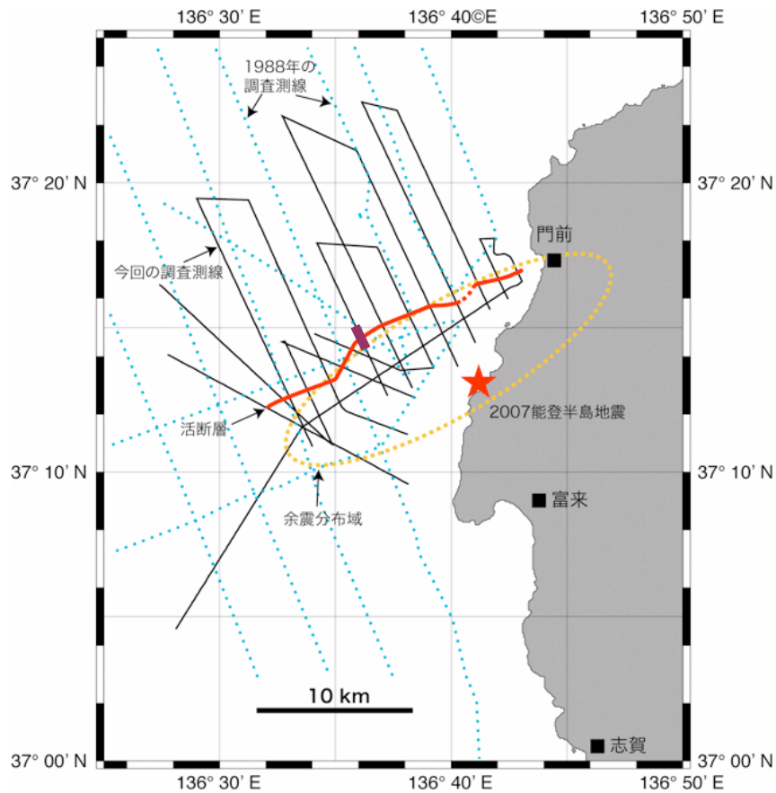
音波探査測線（黒）と断層位置（赤）及び1988年の音波探査測線（青点線）
