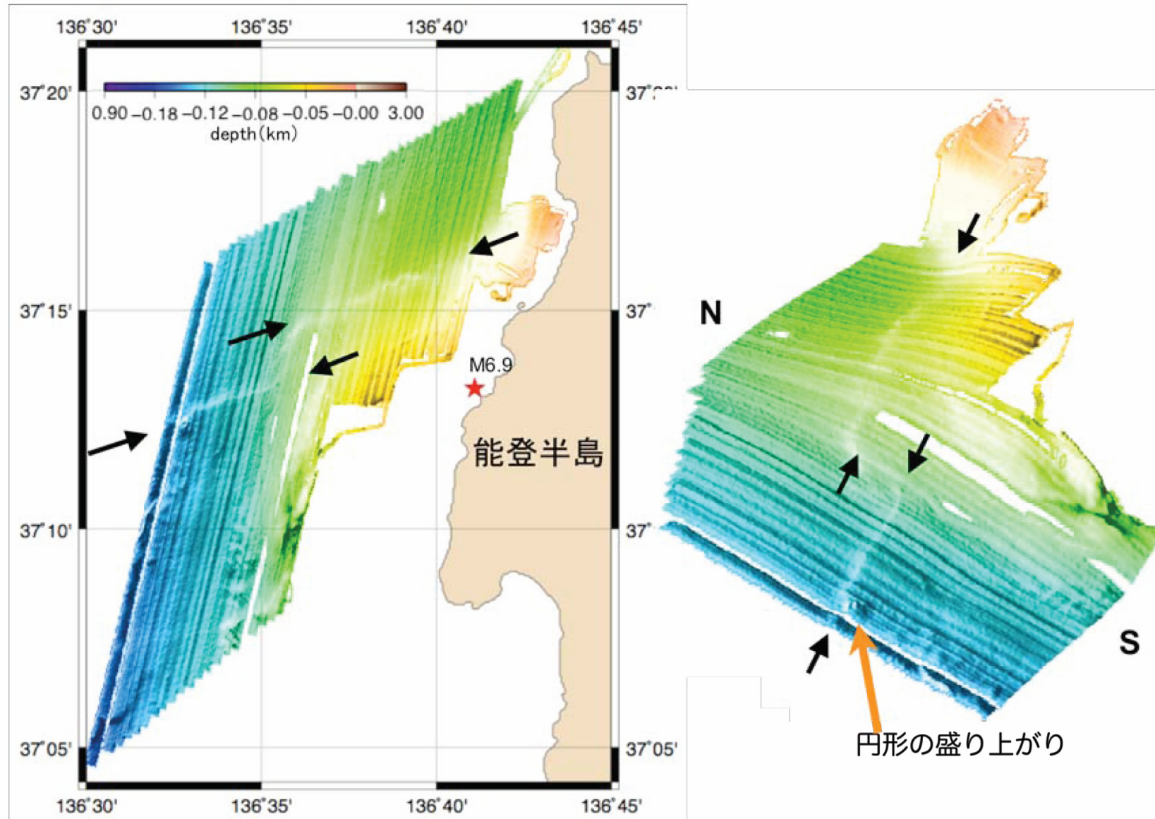
図. 海底地形の陰影図（左）および3次元表示図（右）
