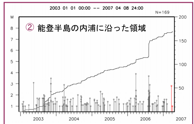
各領域内の地震活動経過図、回数積算図
