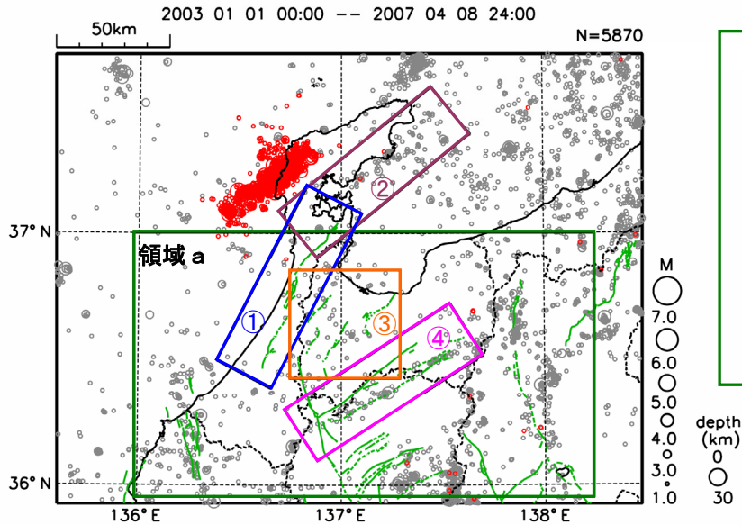
震央分布図 (2003年1月以降、 M \geq 1.0 )
