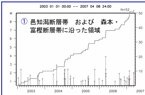
各領域内の地震活動経過図、回数積算図
