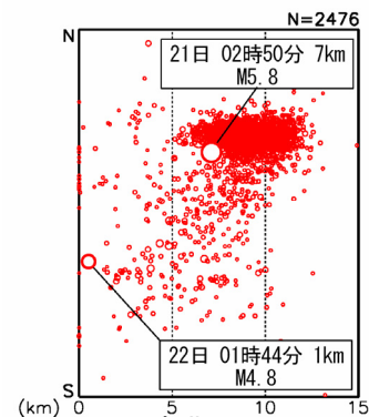
南北断面図
