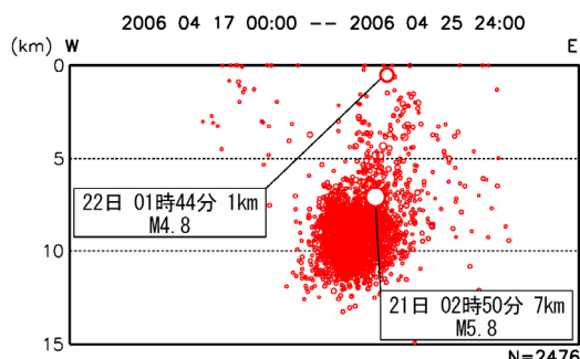
東西断面図
