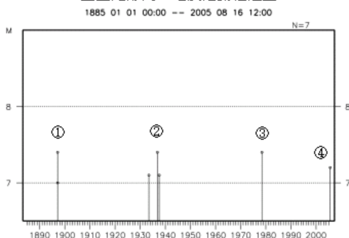
上図矩形内の地震活動経過図
