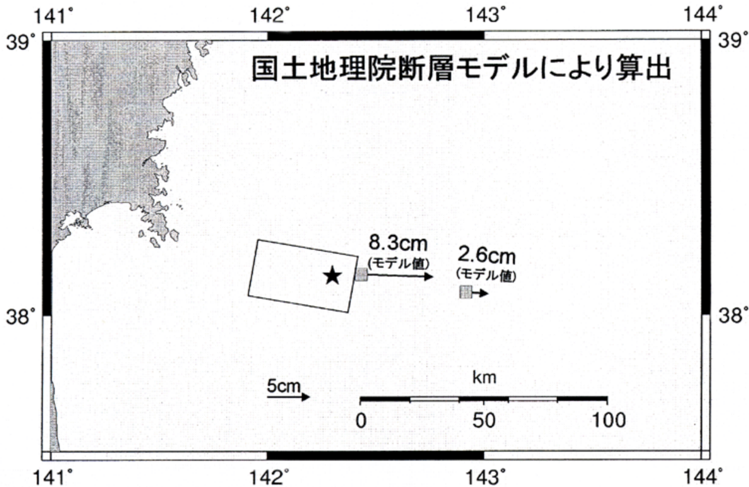
図 3. 国土地理院の断層モデルから計算された 2005 年 8 月 16 日発生地震による地殻変動の水平ベクトル
