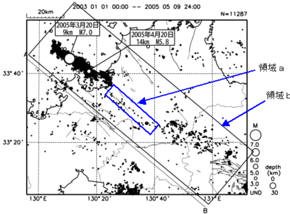
震央分布図（2003年以降、Mすべて）
