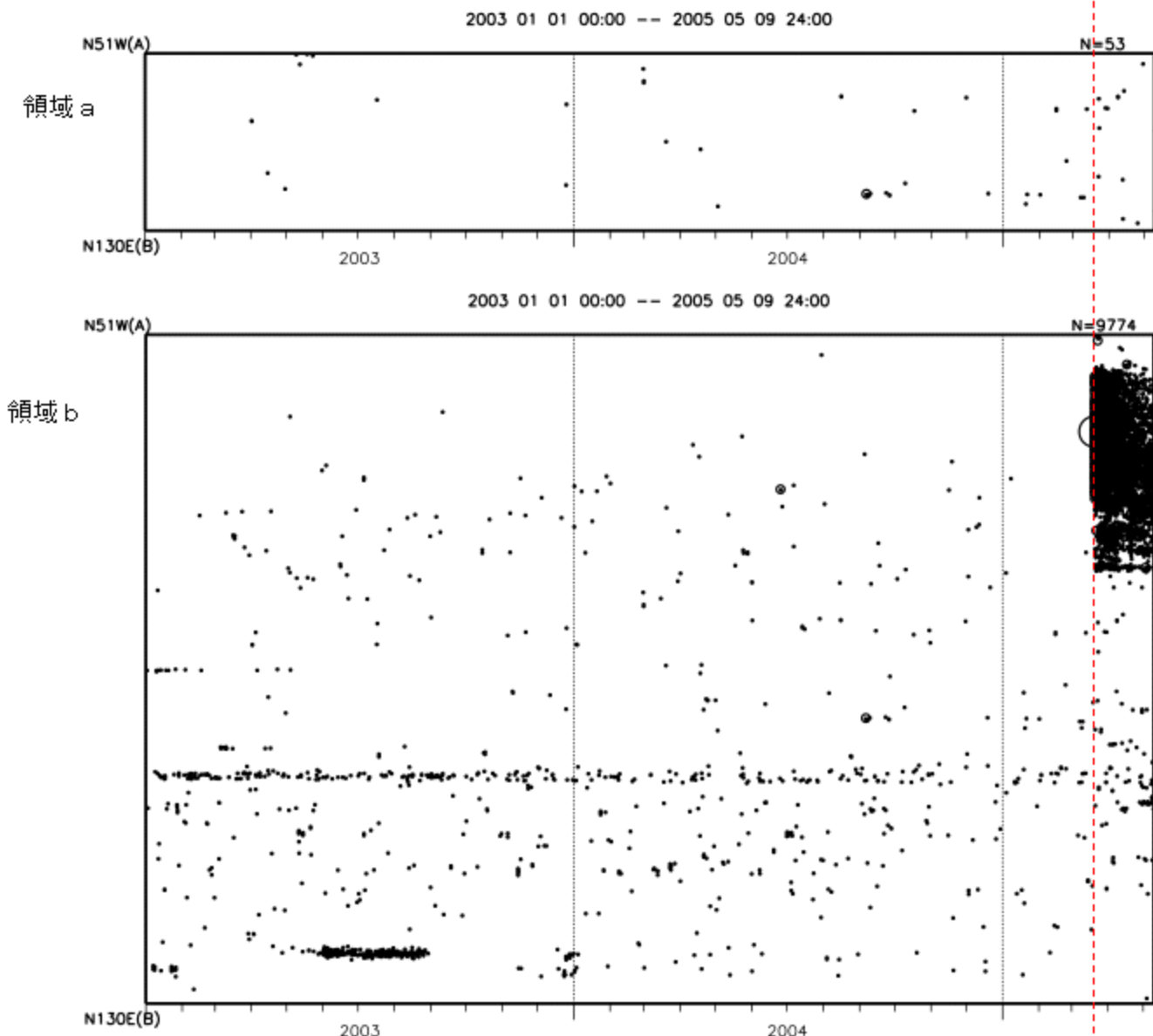
時空間分布図 (A-B 投影)
