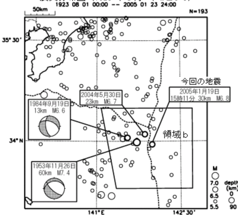
震央分布図（1923年8月～、M≥5.5）
