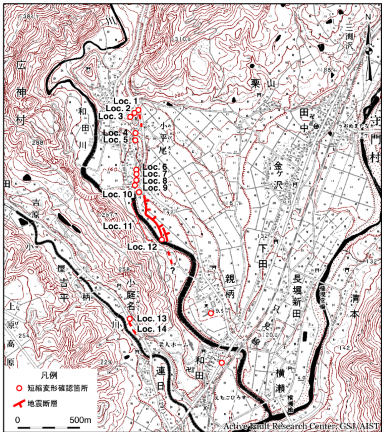
小平尾～小庭名周辺の地表変状分布図
