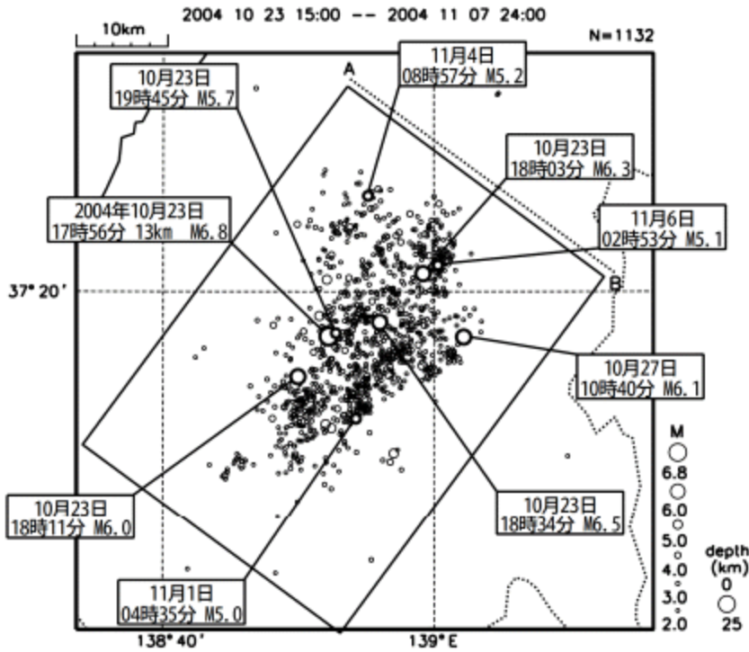
震央分布図（2004年10月23日～、 M \geq 2.0 ）
