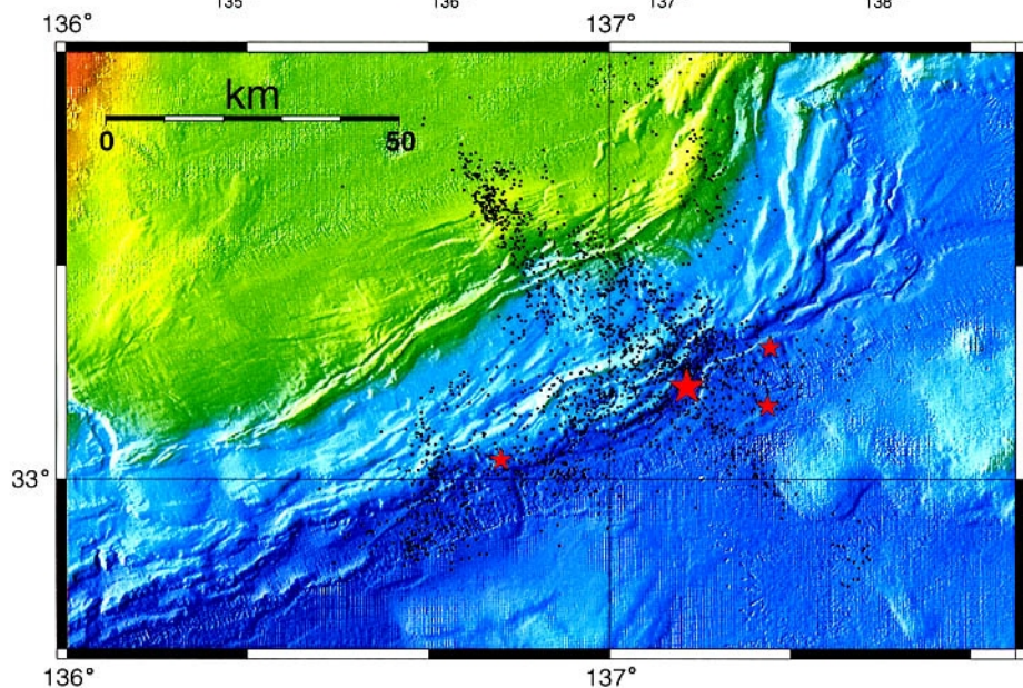
紀伊半島沖の海底地形の陰影図。黒丸は気象庁一元化震源（2004年9月5日19時より4週間）。大きな赤星印は本震，小さな赤星はM6.0以上の震央の位置。
