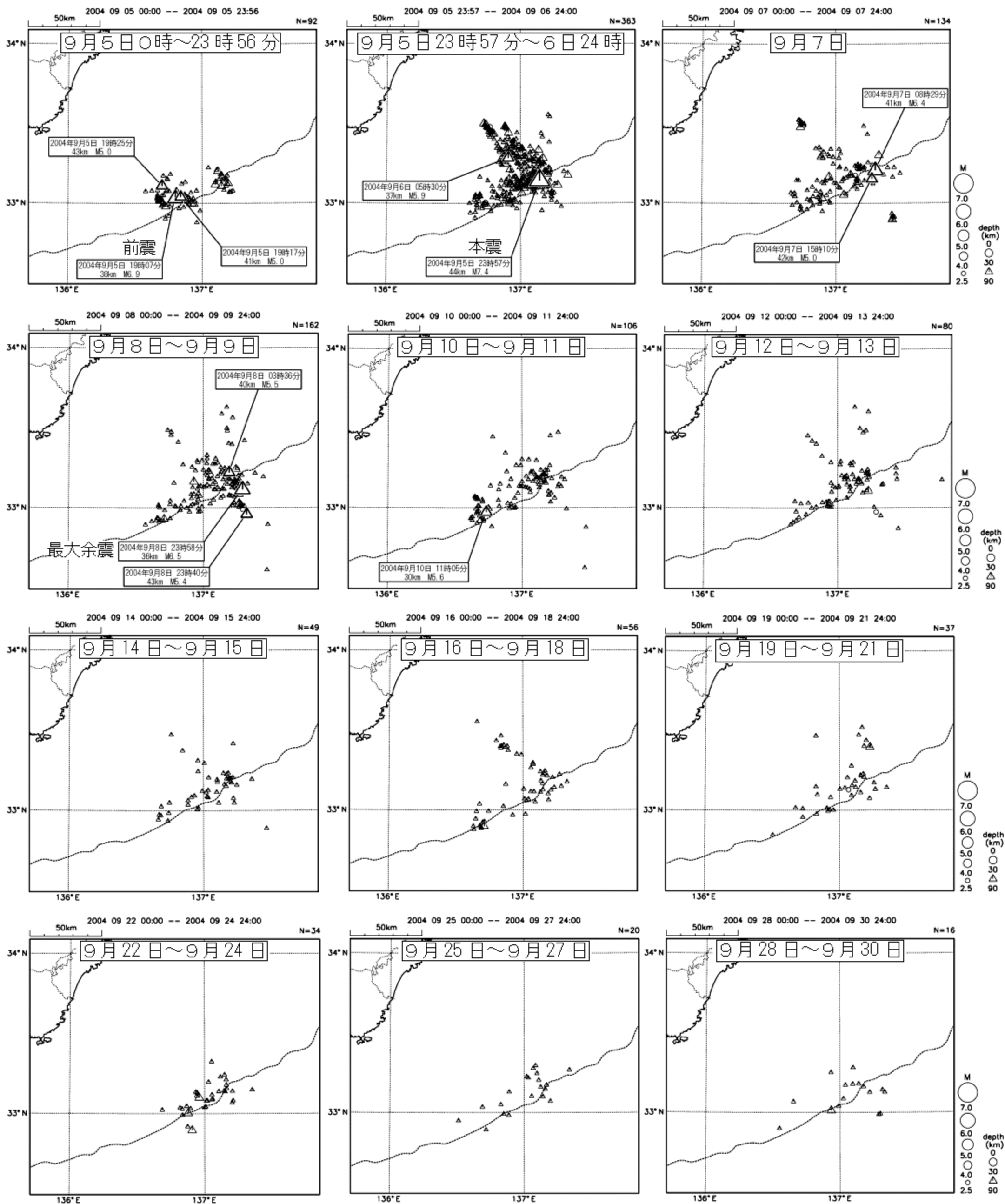
震央分布図（M \geq 2.5）
