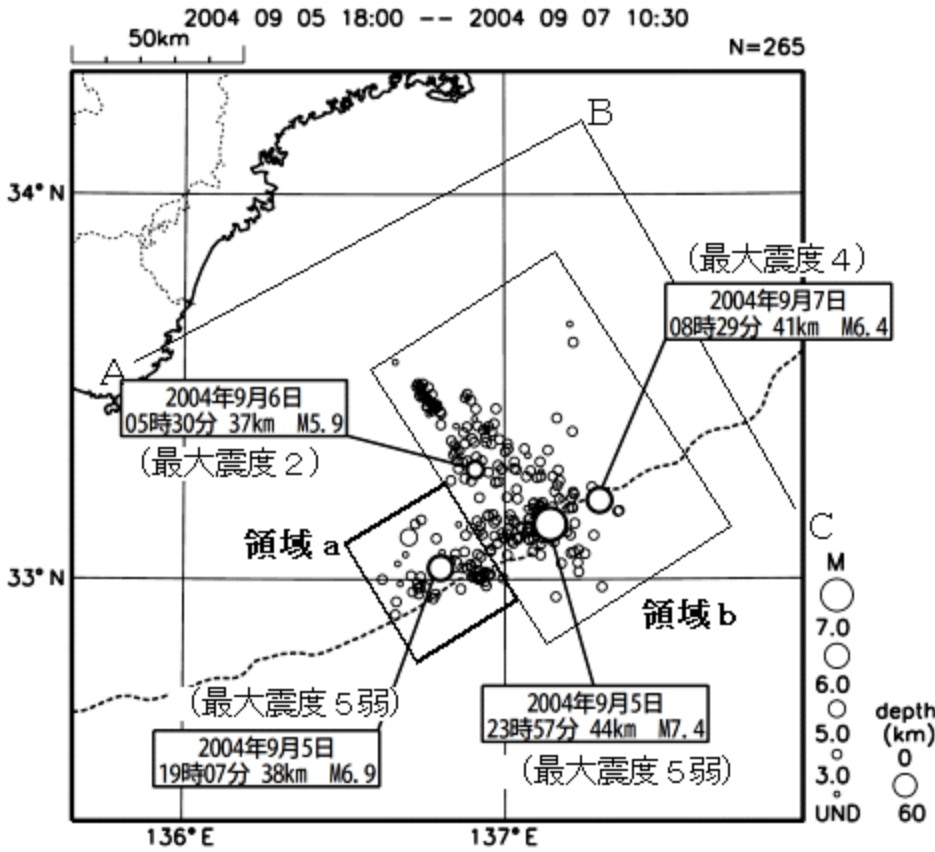
震央分布図（2004年9月5日18時～、Mすべて）
