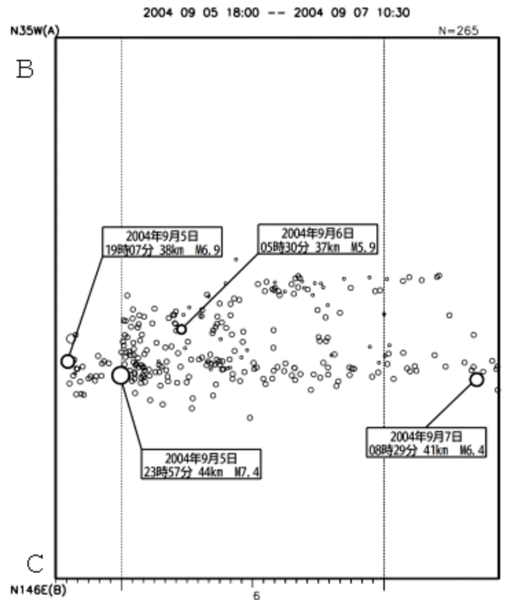
時空間分布図（B-C方向投影）
