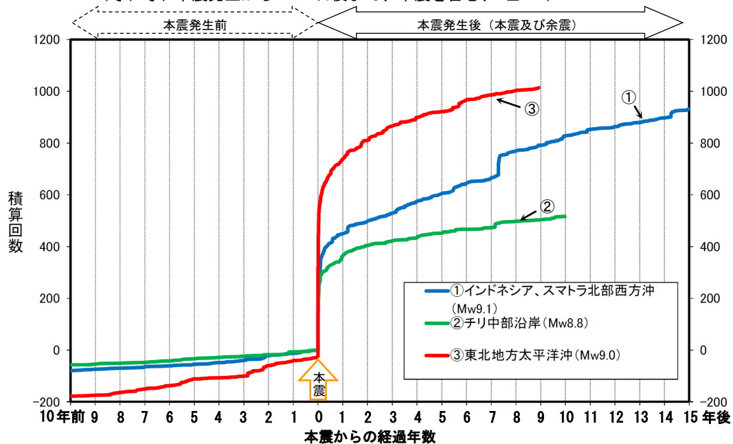
図4-2 世界の海域で発生した主な地震の本震発生前後の地震回数比較 (それぞれ本震発生の10年前から2020年3月11日まで(但し、インドネシア、スマトラ北部西方沖の地震は2019年12月26日まで)、 M \geq 5.0 )
