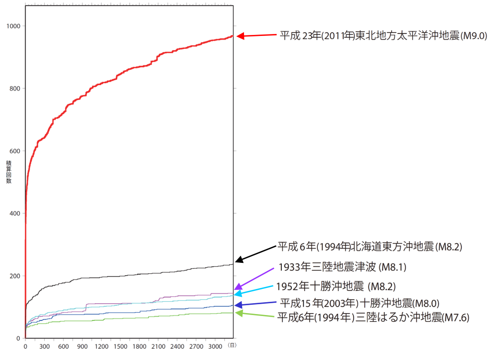
図4-1 日本の海域で発生した主な地震の余震回数比較 (それぞれ本震発生から3288日後まで、本震を含む、 M \geq 5.0 )
