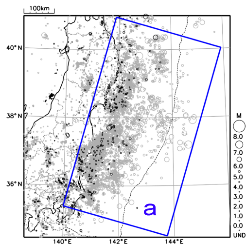
図 1-3 震度 1 以上を観測した地震の震央分布図 （2008 年 3 月 1 日～2020 年 3 月 11 日 14 時 45 分、深さ・M すべて） 東北地方太平洋沖地震の発生から 8 年後（2019 年 3 月 11 日 14 時 46 分） 以降に発生した地震を濃く表示している。 領域 a：東北地方太平洋沖地震の余震域
