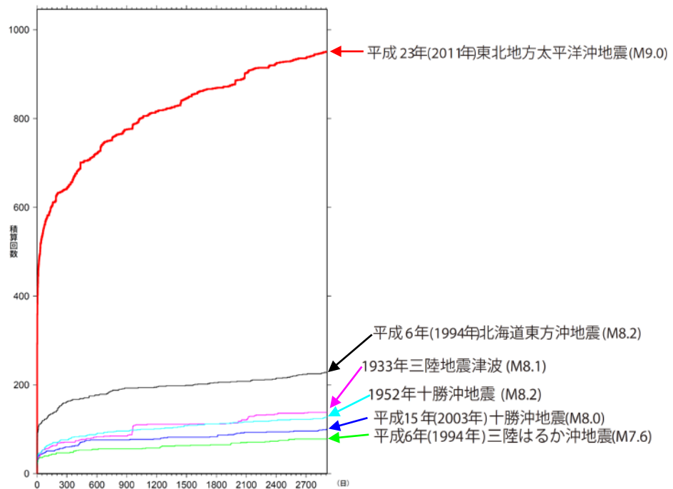
図4-1 日本の海域で発生した主な地震の余震回数比較 (それぞれ本震発生から2911日後まで、本震を含む、 M \geq 5.0 )
