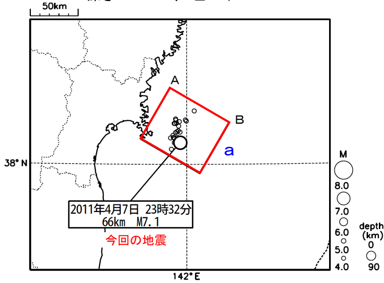
震央分布図(2011年3月9日～2011年4月8日12時、 深さ0～90km、M≥4.0)
