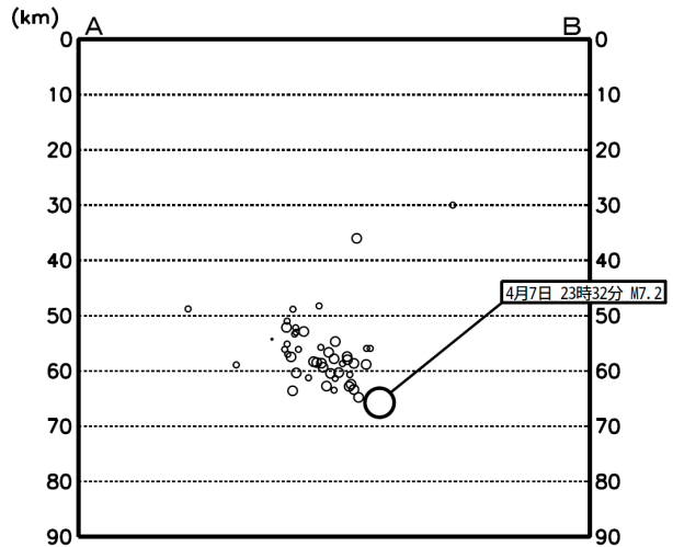
領域a内の断面図 (A-B投影、M全て)
