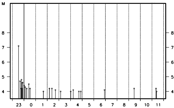
領域a内の地震活動経過図 (4月7日23時から8日12時)
